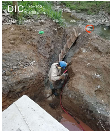
Demolición de roca en descarga del desarenador [Localización:K0+110]
